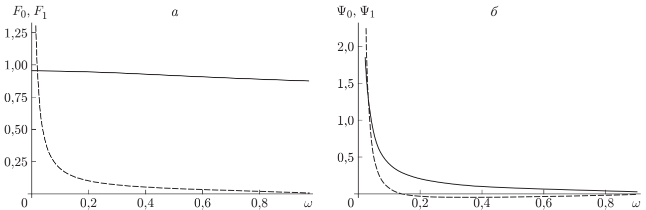
Рис. 1. Зависимости первого F_0 (сплошные линии) и второго F_1 (штриховые линии) приближений вертикальной (а) и горизонтальной (б) скоростей ВГВ от частоты \omega при z = -1,2 , y = 0,8
