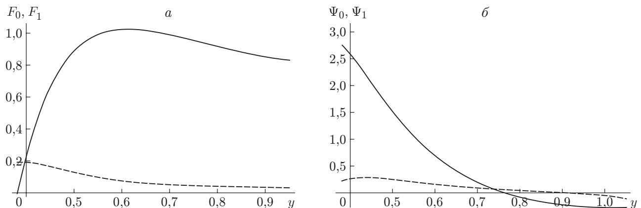
Рис. 2. Зависимости первого F_0 (сплошные линии) и второго F_1 (штриховые линии) приближений вертикальной (а) и горизонтальной (б) скоростей ВГВ от горизонтальной координаты y при z = -1,2 , \omega = 0,5
