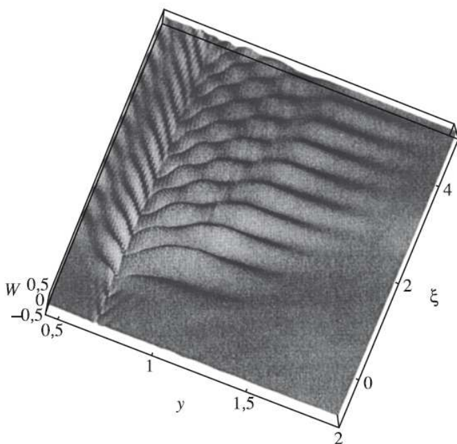
Рис. 1. Внутренние волны в океане переменной глубины.
